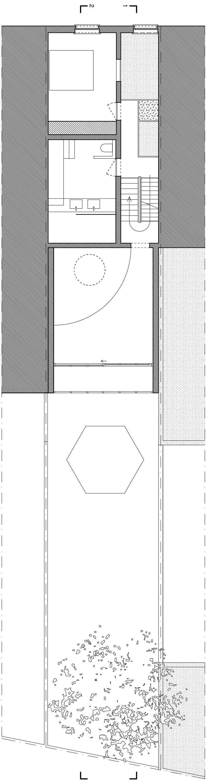
VERDIEPING 1
