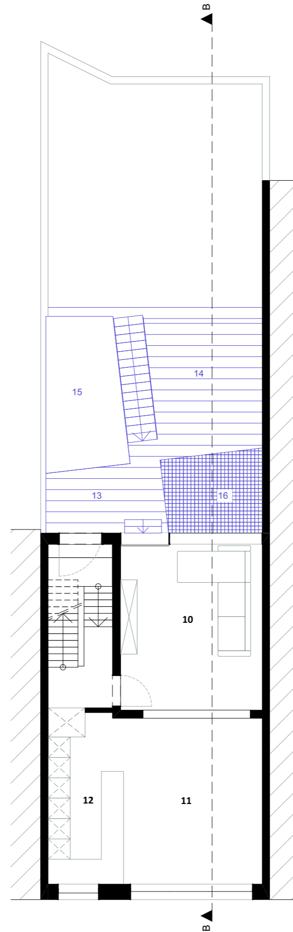
PLAN VERDIEPING 1 10. ZITRUIMTE / 11. EETRUIMTE / 12. KEUKEN / 13. DAKTERRAS / 14. DAKTERRAS / 15. GROENDAK / 16. VIDE
