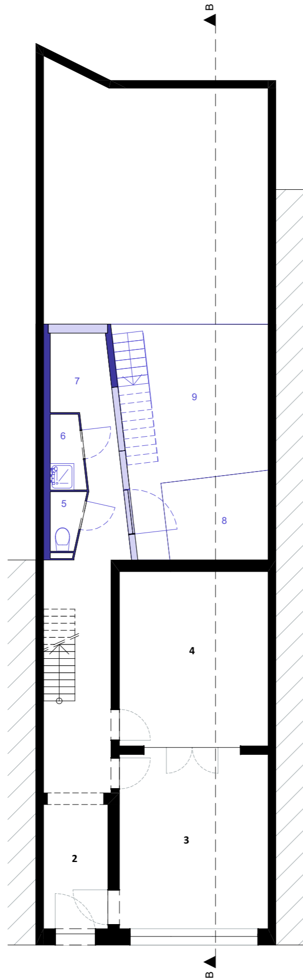
PLAN BEGANE GROND 2. INKOMHAL / 3. PRAKTIJKRUIMTE OF BUREAU / 4. PRAKTIJKRUIMTE OF BUREAU / 5. TOILET / 6. DOUCHE / 7. KEUKEN / 8. PATIO / 9. OVERDEKT TERRAS
