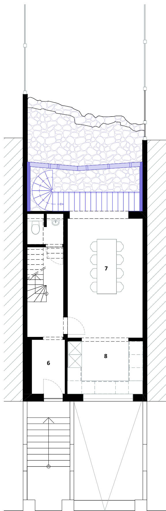
PLAN BEGANE GROND 6. INKOMHAL / 7. LEEFRUIMTE / 8. KEUKEN
