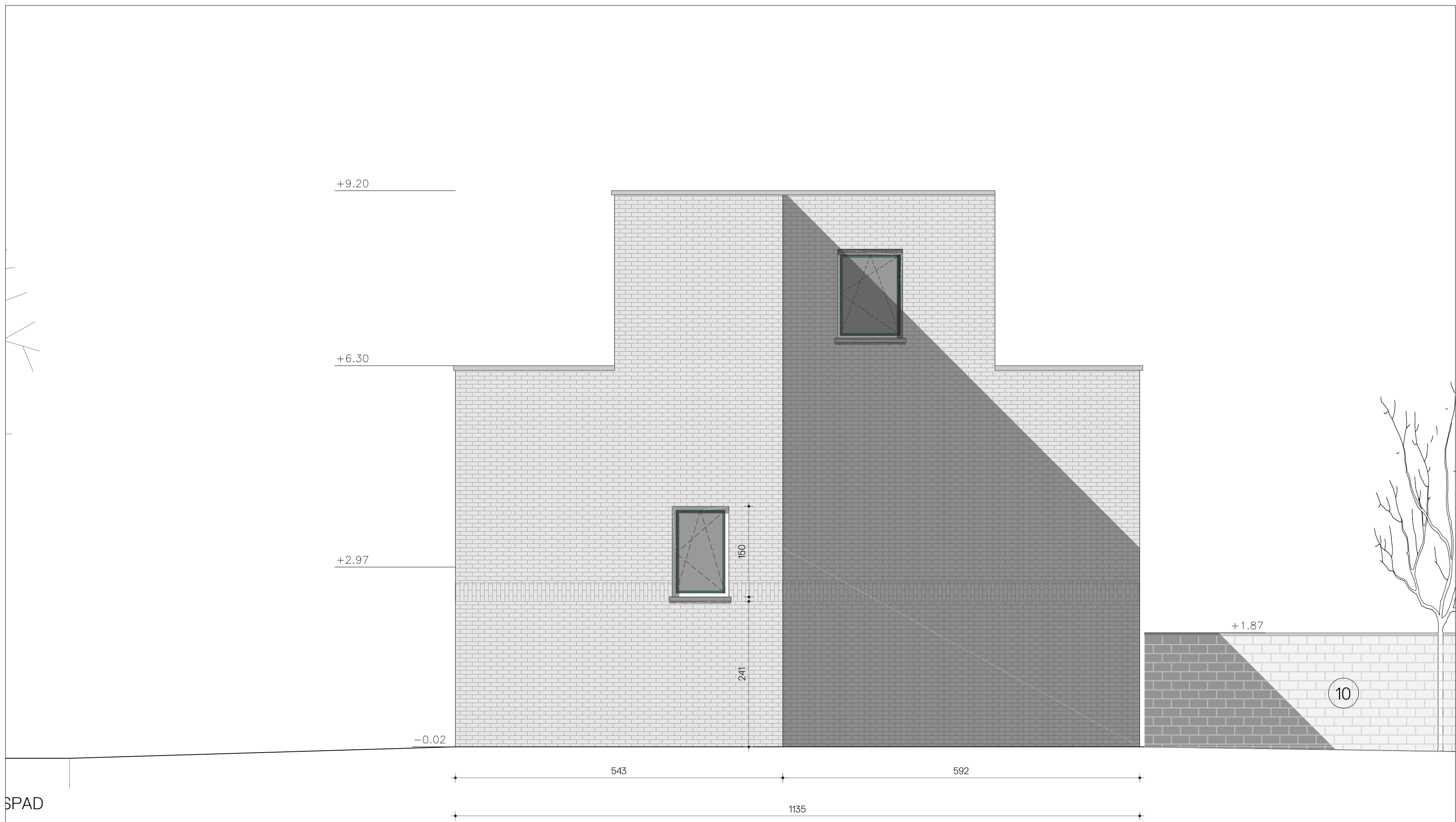
AANZICHT ZIJDE PARKING
