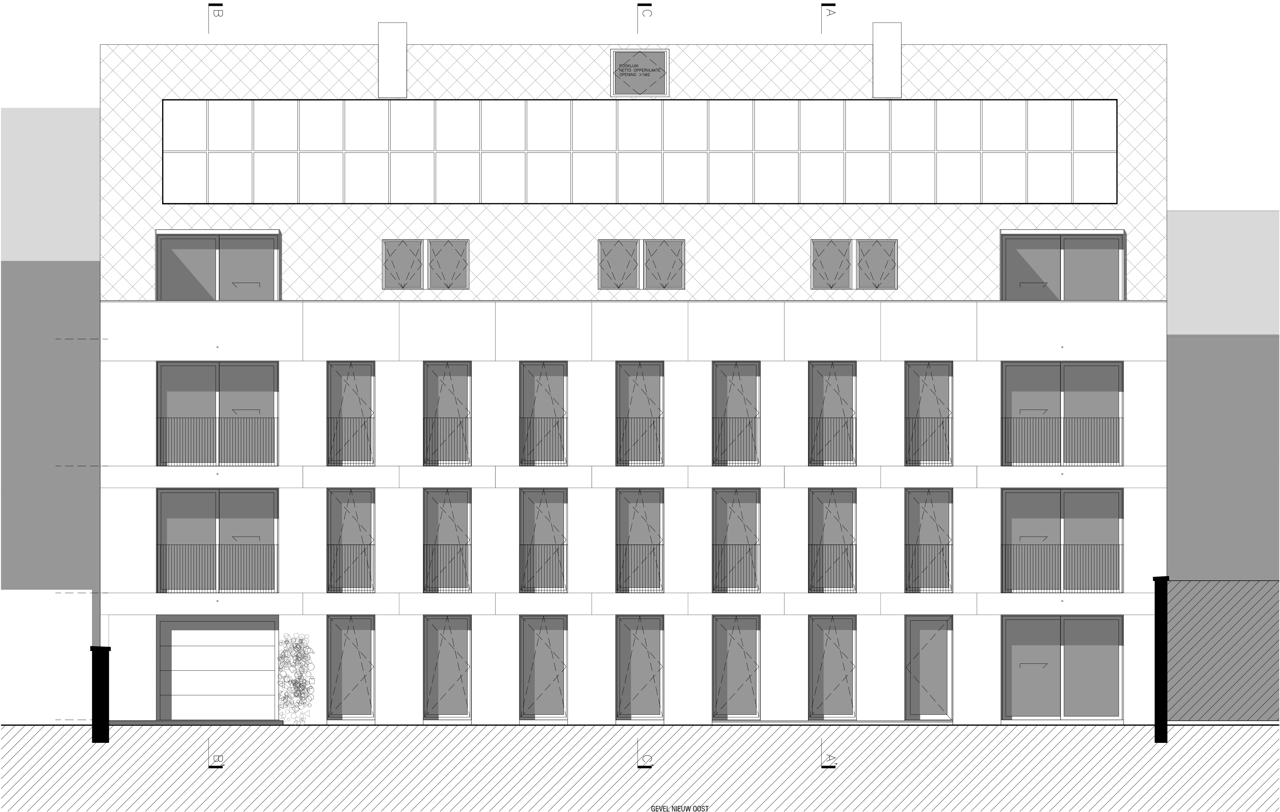
GEVEL NIEUW OOST
